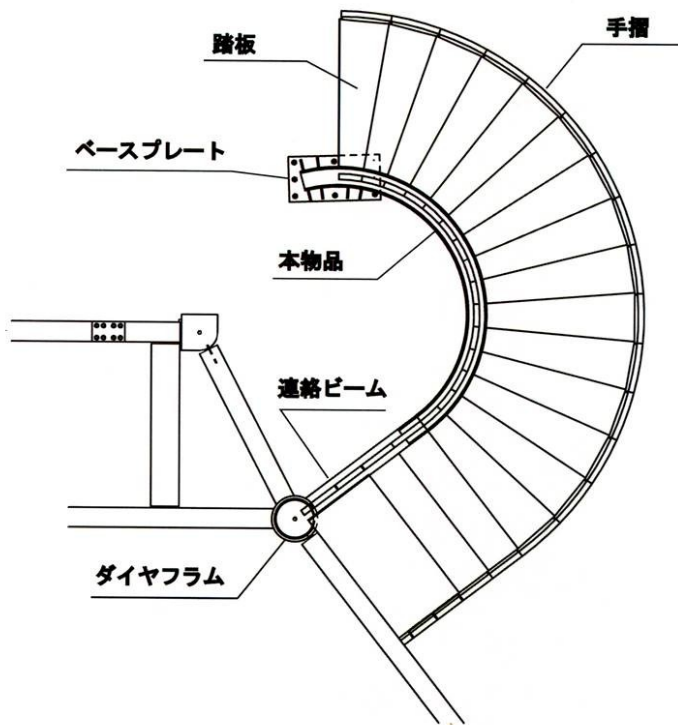
【使用状態の参考平面図】
